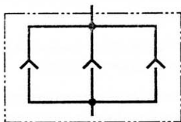
Рисунок 5а — Три независимых соединительных элемента
