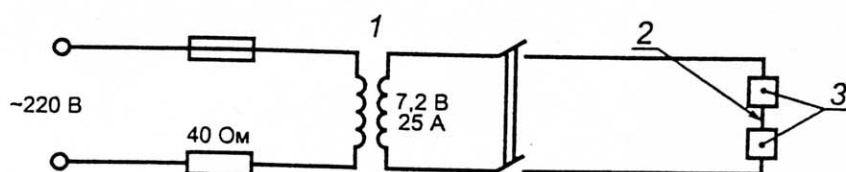
Рисунок В.7 — Устройство для подготовки вольфрамовых проволочек методом оплавления
