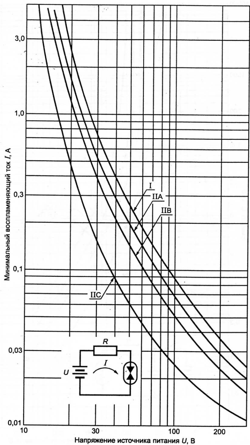
Рисунок А.1 — Омические цепи
