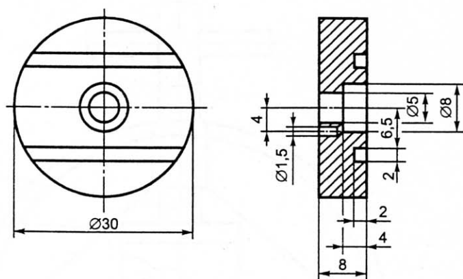
Рисунок В.2 — Кадмиевый контактный диск
