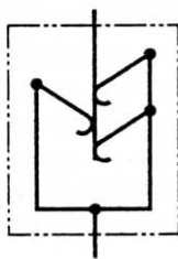
Рисунок 5b — Три соединительных элемента, не являющихся независимыми
