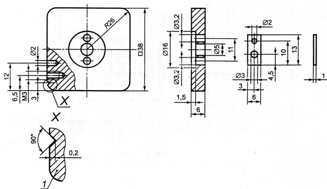
Рисунок В.3 — Держатель проволочек
